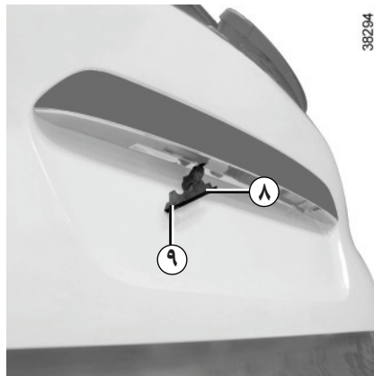
چراغ پلاک ۸ - چراغ ۸ را با فشار دادن زبانه ۹ آزاد کنید. - برای دسترسی به لامپ روکش را بردارید. نوع لامپ: W5W.
