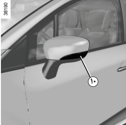
چراغ راهنمای جانبی ۱۰ به دلیل لزوم باز کردن آینه جانبی، به نمایندگی مجاز رجوع کنید. نوع لامپ: W5W.
