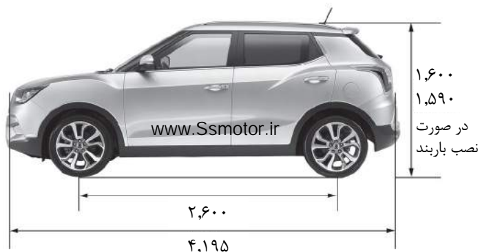
نمای جانبی
